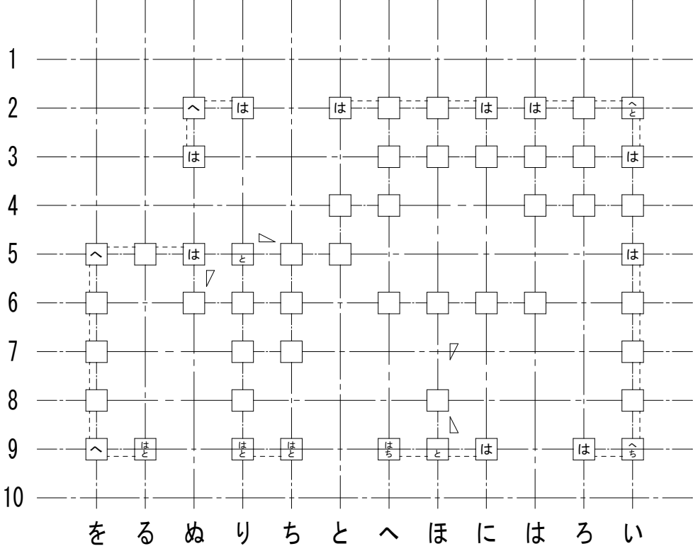
2階柱壁伏図
