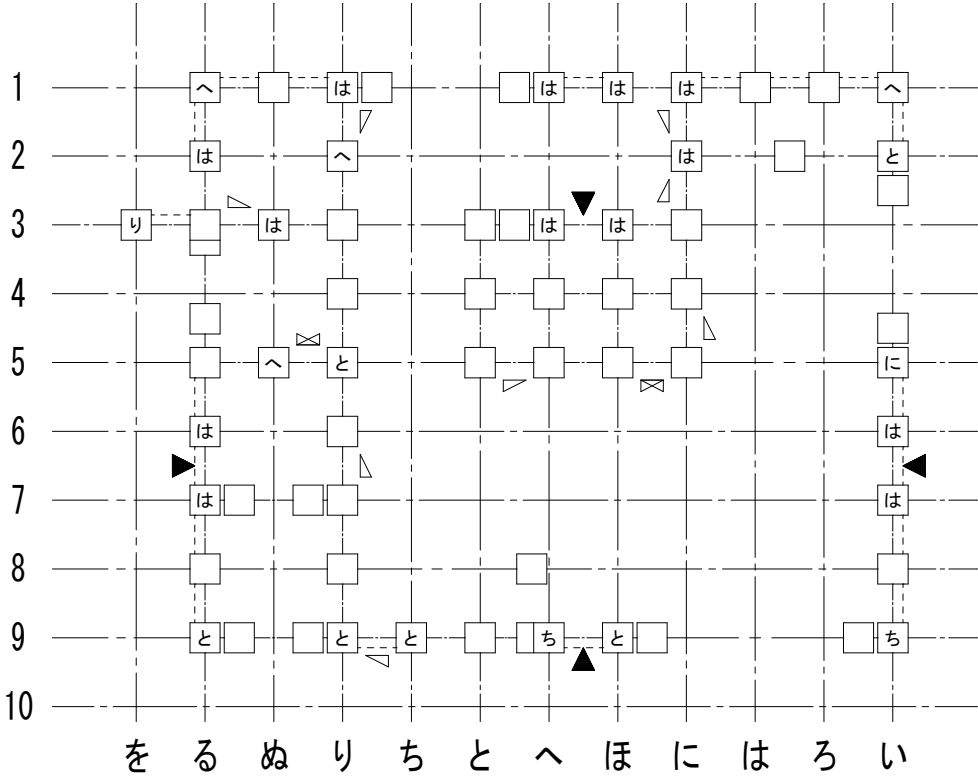
1階柱壁伏図
